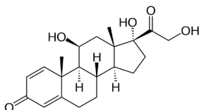
Strukturformel Prednisolon
